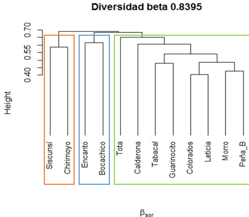
Figura 3. Dendrograma para la agrupación de los lagos con base en la disimilitud en la composición de géneros.
