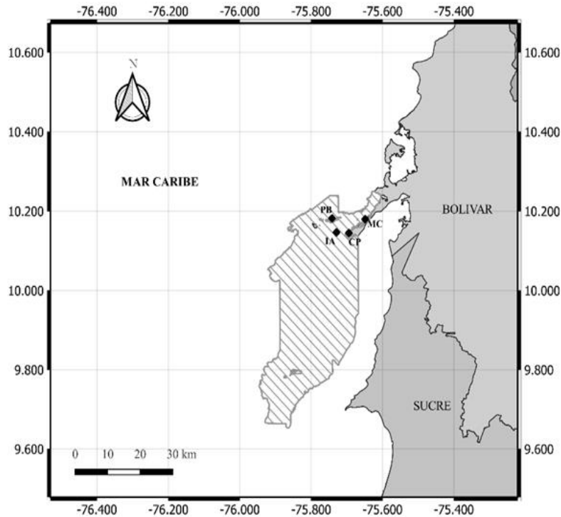
Figura 1. Ubicación del Parque Nacional Natural Corales del Rosario y de San Bernardo (área sombreada), donde se señalan las estaciones de muestreo (PB: Punta Brava, IA: Isla Arena, MC: Mojaculo, CP: Ciénaga El Pelao).
