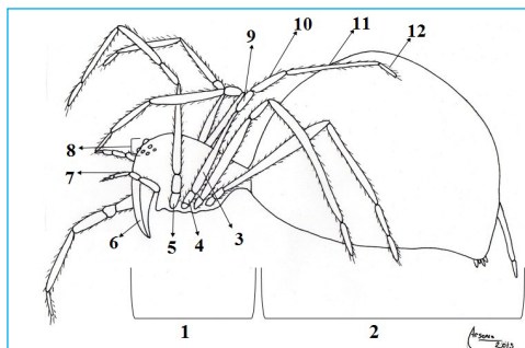
Fig. 1. Esquema de la morfología de un arácnido. 1) Prosoma; 2) Opistosoma; 3) Fémur; 4) Trocánter; 5) Coxa; 6) Quelicero; 7) Pedipalpo, 8) Ojos simples; 9) Rotula; 10) Tibia; 11) Metatarso; 12) Tarso.
