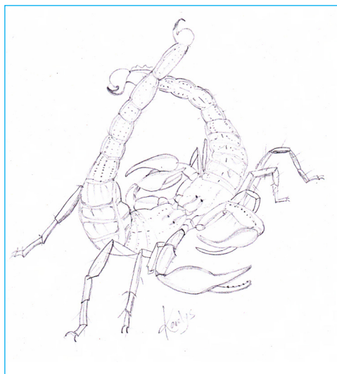
Fig. 5. Escorpiones en danza de apareamiento.
