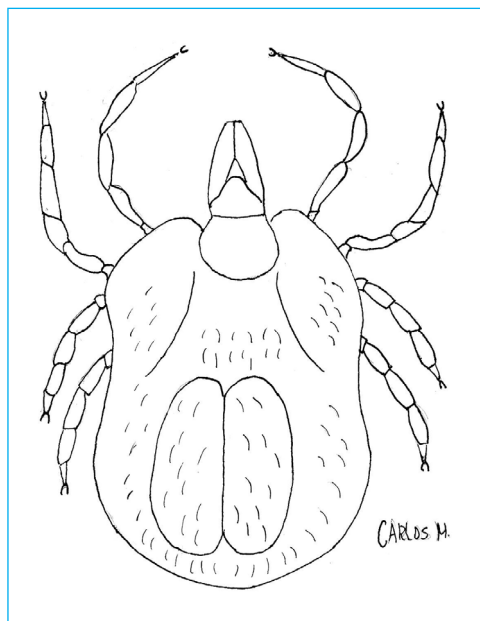
Fig. 7. Esquema general de un ácaro.
