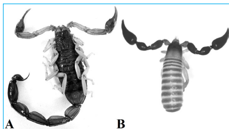
Fig. 10. Familias de arácnidos. A) Buthidae, B) Olpiidae.
