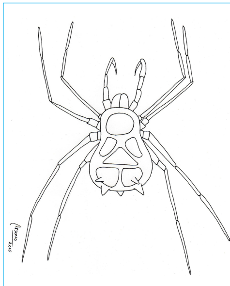
Fig. 6. Esquema general de un opilión.
